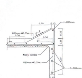
แปลนรายละเอียดอาคารสาขาย่อยที่งานหน้า มาตราส่วน 1:50
