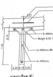
รายละเอียด (8) มาตราส่วน 1:20
