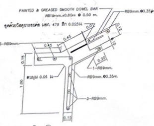
รายละเอียด (7) มาตราส่วน 1:20
