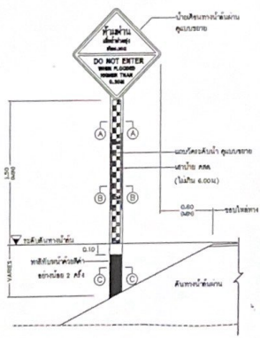
แสดงการติดตั้งเสาป้ายเตือนทางน้ำล้นผ่าน มาตรฐาน 1:20
