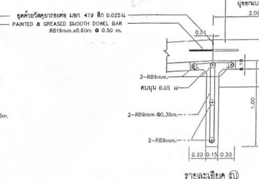
รายละเอียด (9) มาตราส่วน 1:20
