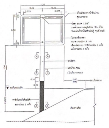
แสดงการติดตั้งเสาป้ายเตือนทางลดระดับ มาตรฐาน 1:25
