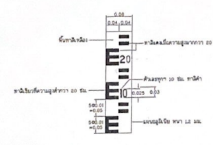
แบบขยายแผนบริดระดับน้ำ ไม่แสดงทิวทัศน์
