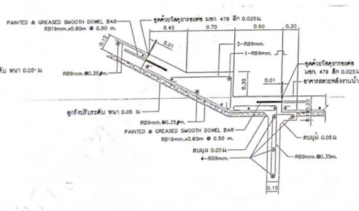
รายละเอียด (4) มาตราส่วน 1:20
